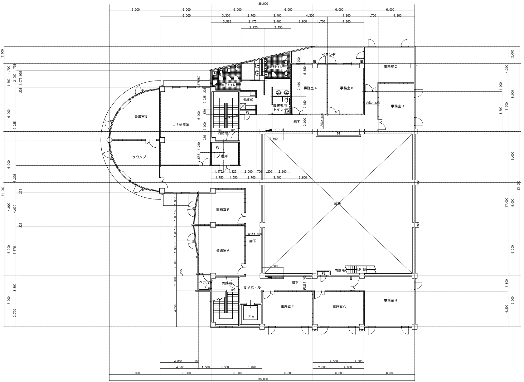
3 階平面図
